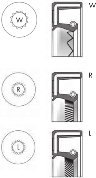
螺旋回流纹的多种设计
