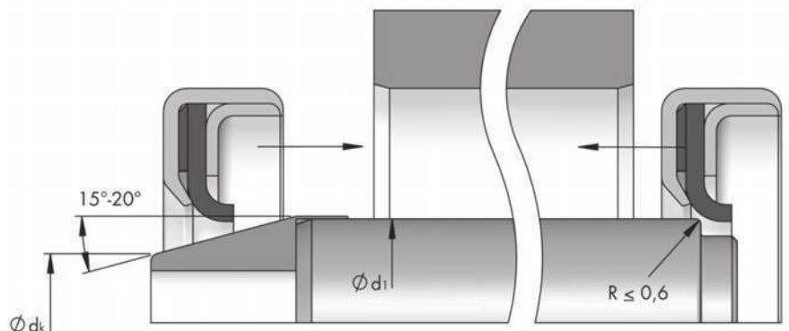
安装锥套 WCP21
