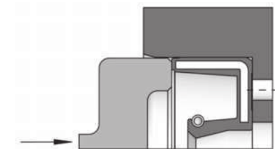
用于旋转油封的多种安装工具
