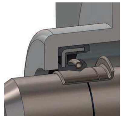
旋转油封与WASH R 轴套的配合
