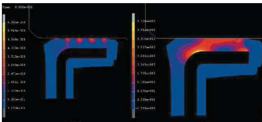
使用有限元法模拟座孔的静密封
