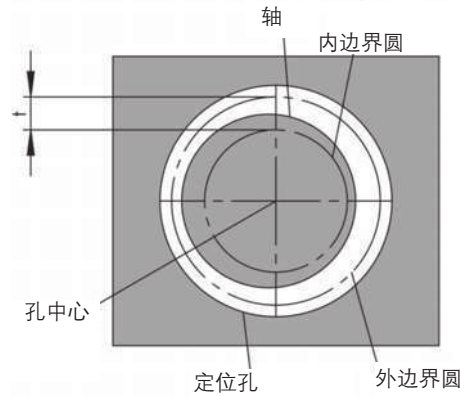
不圆度公差说明
