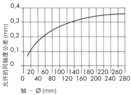
安装座孔和旋转轴之间允许的同轴度公差
